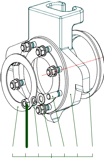
Anschluss / connection / connexion DN 100
